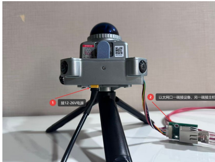
外置以太网口接线图
